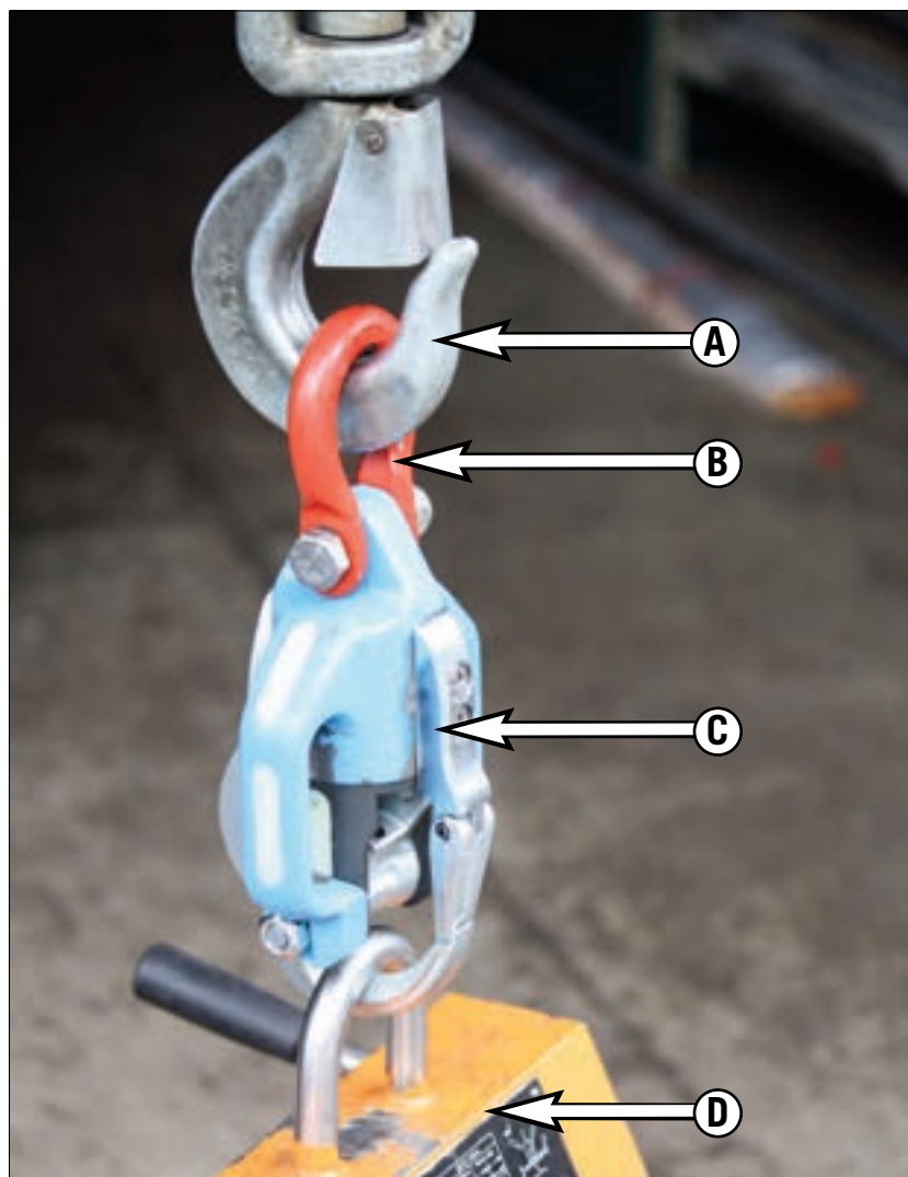
Mode d'attache : « Traction par manille/alésage »
