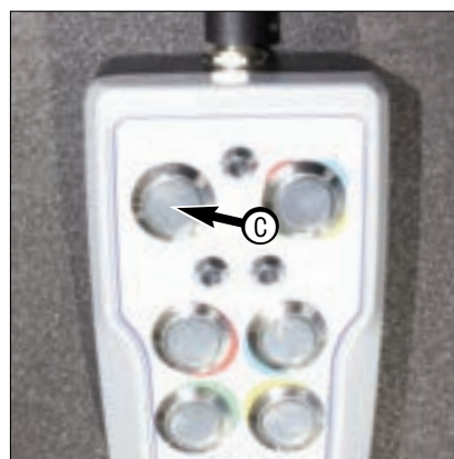
2) La charge peut maintenant être libérée: appuyer sur le bouton C et dans un délai de 0,5 s ...
