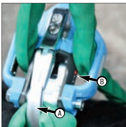
1) Abaisser la charge jusqu'à avoir une traction max. de 10 kg sur le crochet A du LUDWIG HOOK (la DEL B du LUDWIG HOOK s'allume).
