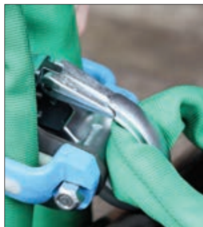
4) Vérifier la sécurité du verrouillage ! La charge peut maintenant être levée.
