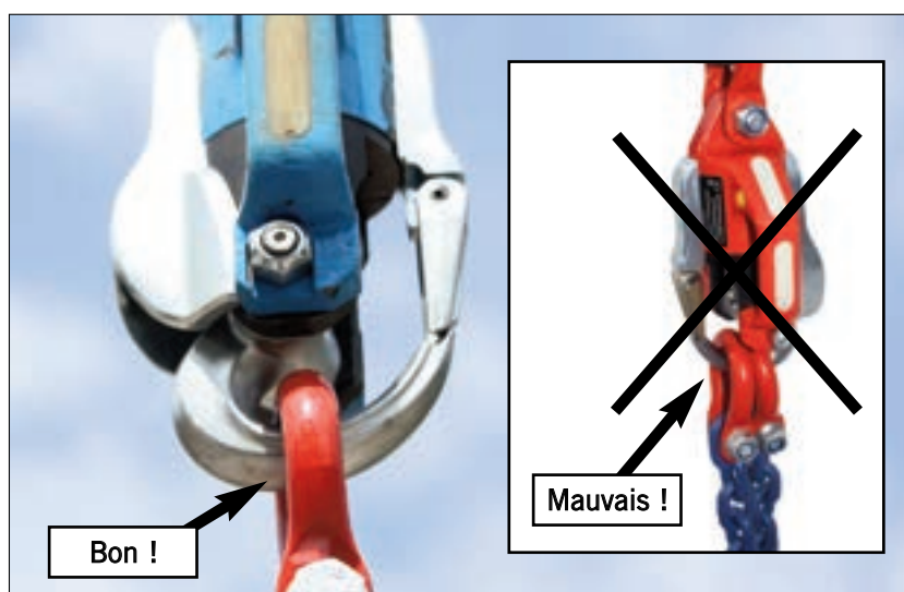
Point d'attache correct (petite image : point d'attache incorrect)
